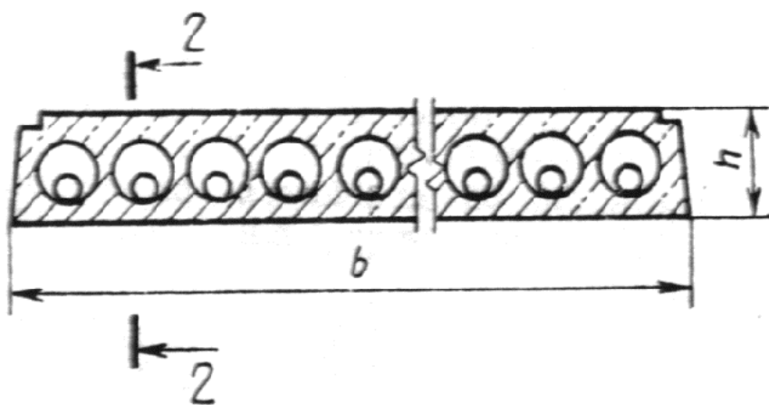
Черт. 1 Плита типа 4ПК 1-1
