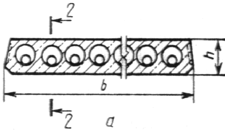
Плиты типов 1ПКТ, 2ПКТ, 3ПКТ
