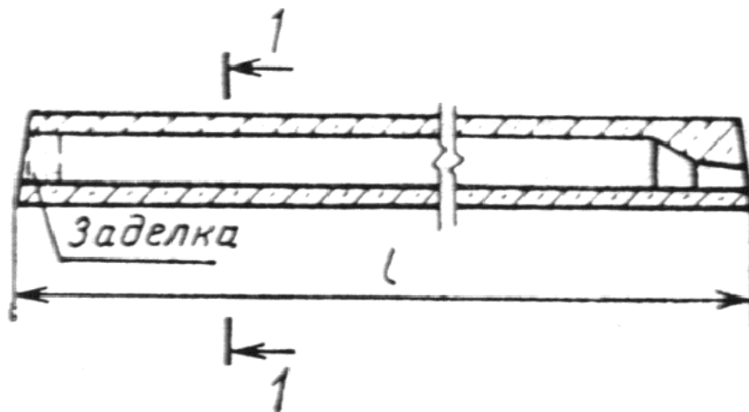
Черт. 1 Плита типа 4ПК 1-1
