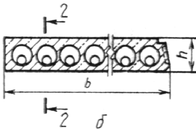
Плиты типов 1ПКК, 2ПКК, 3ПКК
