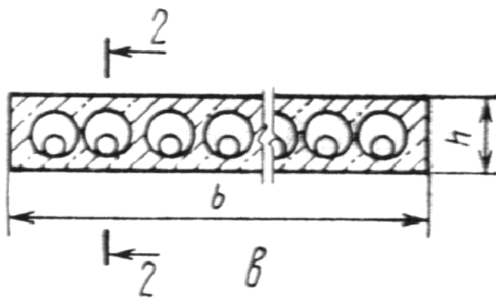
Плиты типов 1ПКК, 2ПКК, 3ПКК
