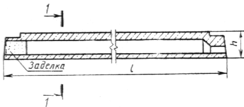
Черт. 2 Плита типа ПГ 1-1
