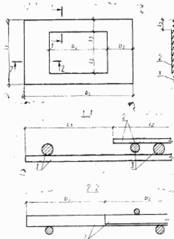
1—нижняя сетка марки Н; 2—верхняя сетка марки В; 3—рабочая арматура
