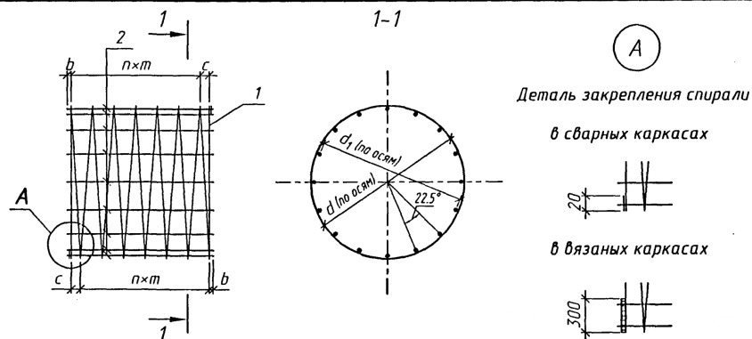
Спецификация элементов на каркас
